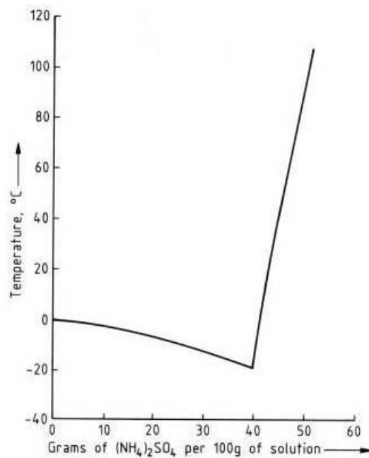
شکل 1-2- نمودار تغییرات انحلال سولفات آمونیوم در آب بر حسب درجه حرارت [2]
