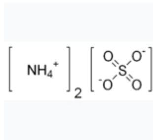
شکل 1-1- ساختار شیمیائی مولکول آمونیوم سولفات
